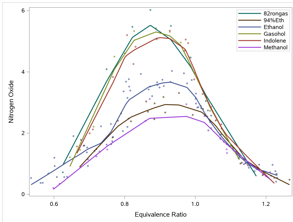
Output 23.6.11 Grouped Loess Fit Plot
