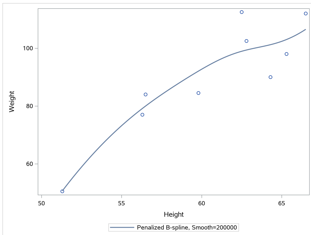
Output 23.6.7 Manually Set Smoothing Parameter
