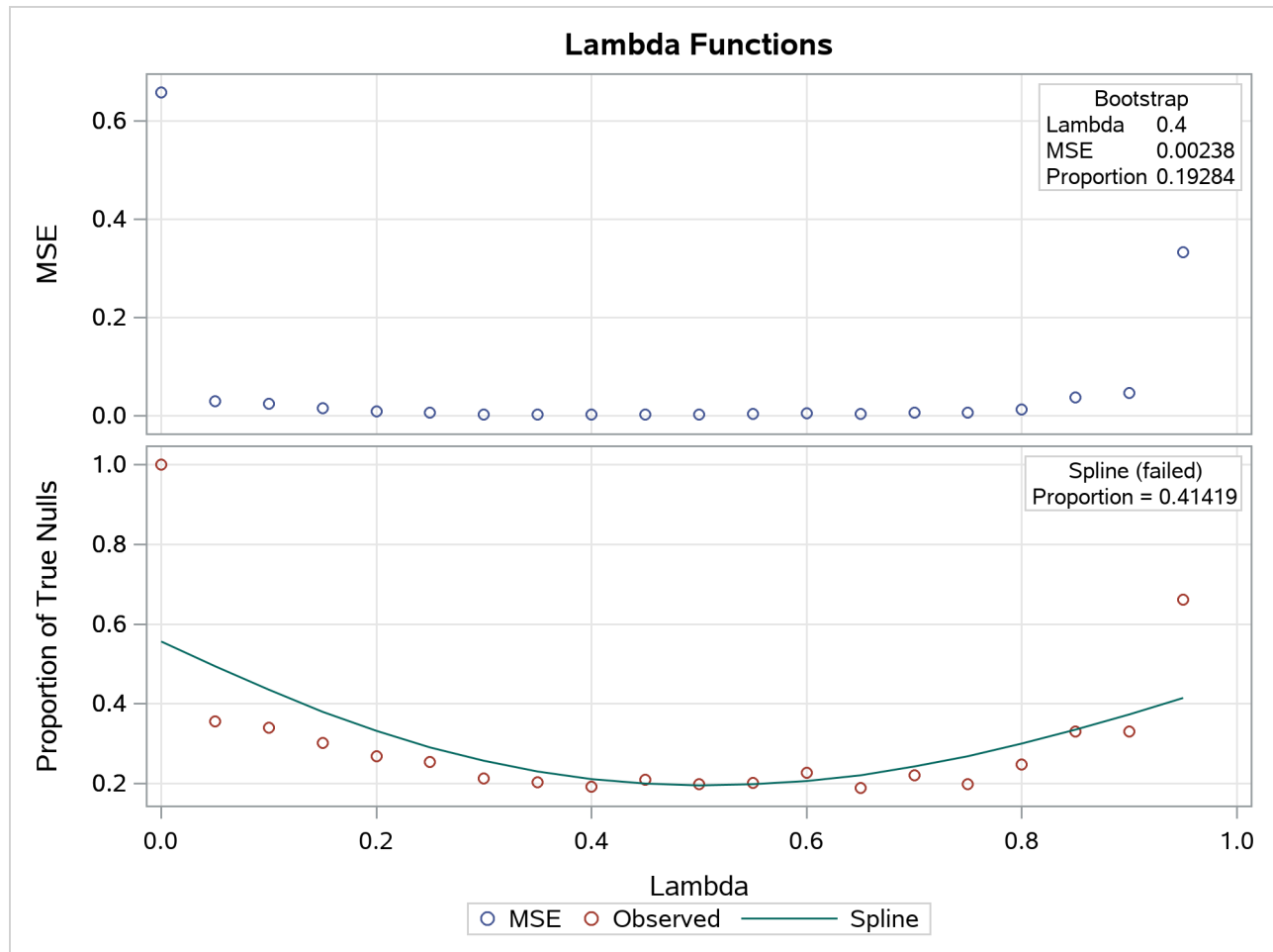
Output 85.6.2 Tuning Parameter Plots
