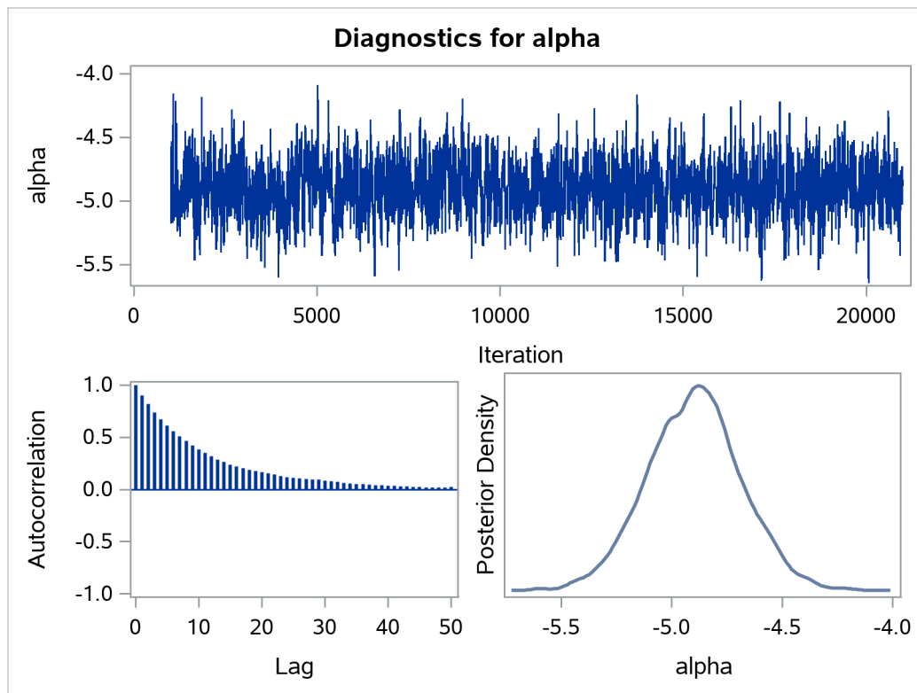
Output 79.6.1 Plots for Parameters
