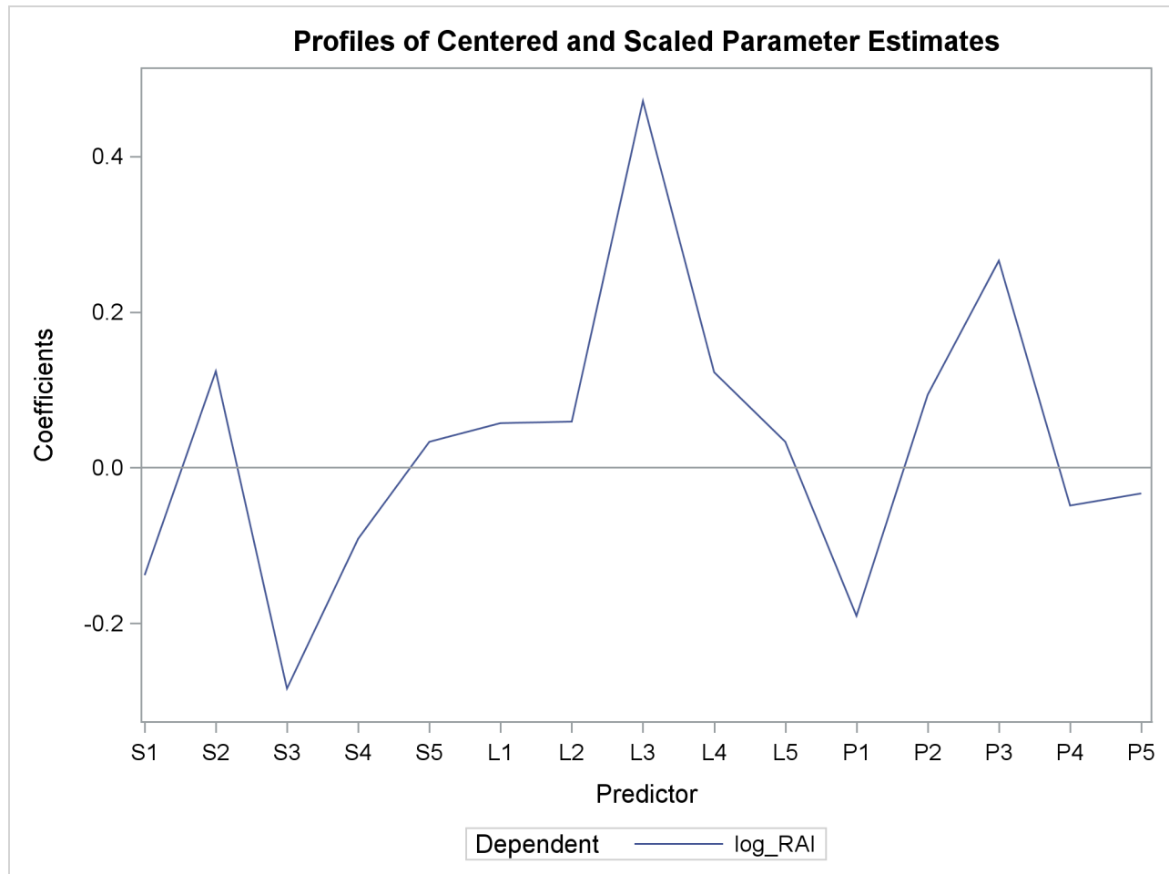
Output 89.1.6 Regression Parameter Profile
