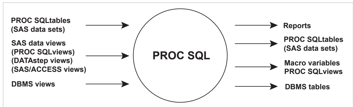
図 7.1 PROC SQL の入力と出力
