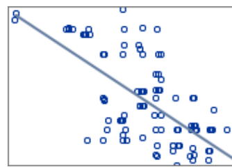
JITTER Specified
