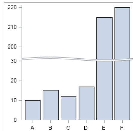
RANGES Specified
