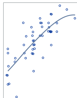
JITTER Specified
